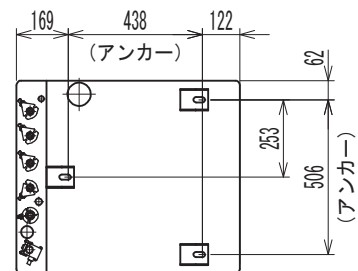
【アンカーボルト位置上面透視図】
