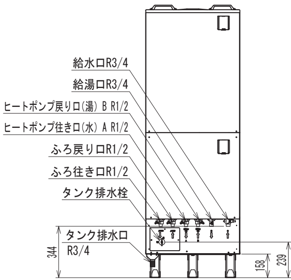
【機器正面図】
