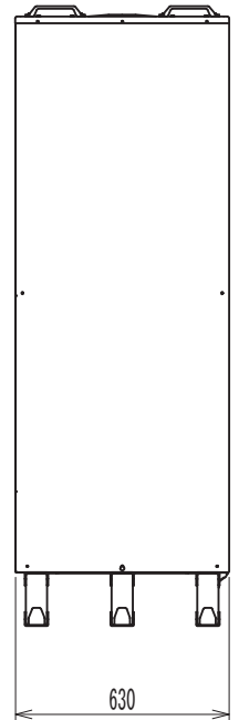
【機器背面図】
