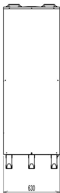
【機器背面図】
