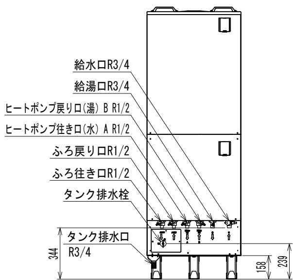
【機器正面図】
