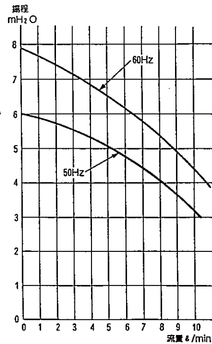
機外揚程線図 (付属の2口ヘッダーを取りはずした場合)
