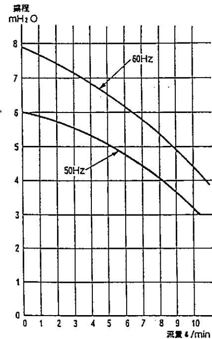
機外揚程線図 (付属の2口ヘッダーを取りはずした場合)
