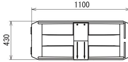
【機器上面図】
