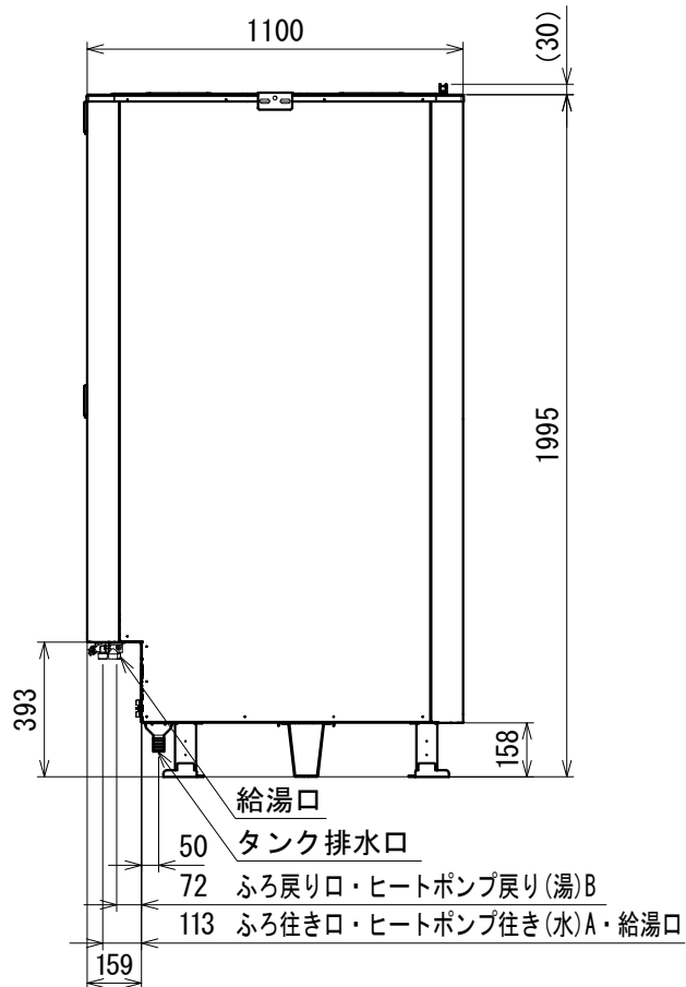
【機器側面図】
