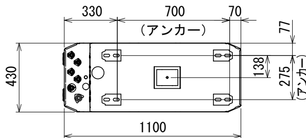
【アンカーボルト位置上面透視図】
