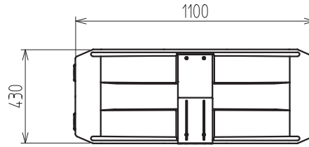
【機器上面図】
