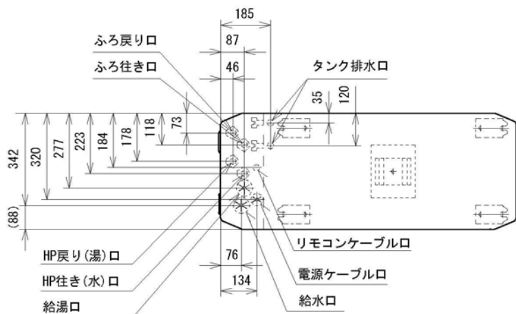
【配管位置図】
