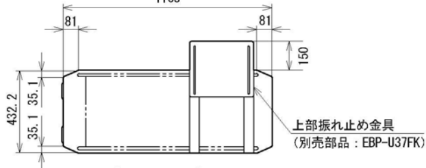
【機器側面図】 1100
