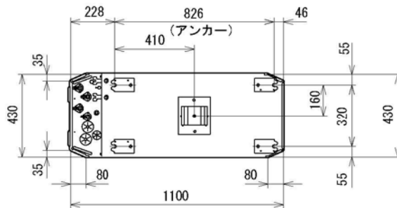
【上面透視図】
