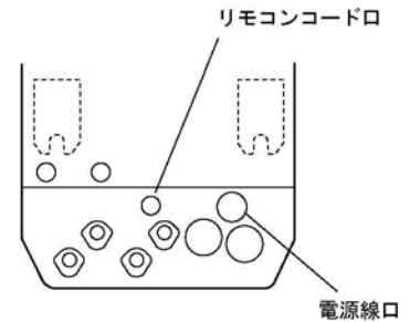
配線取出口 (上面図)
