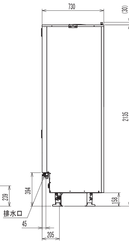
【機器側面図】
