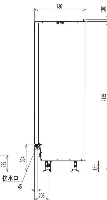
【機器側面図】
