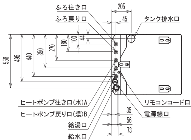
【配管位置図(上面透視図)】
