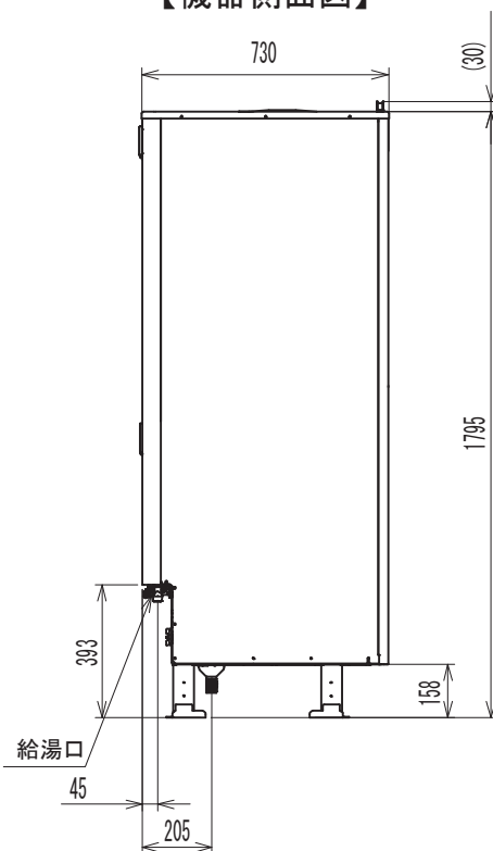
【機器側面図】
