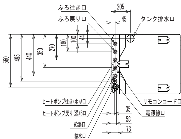
【配管位置図(上面透視図)】
