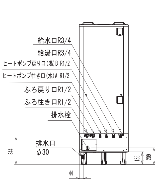
【機器正面図】
