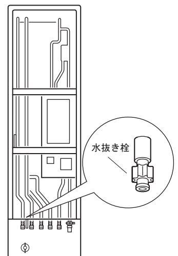
貯湯タンクユニット
