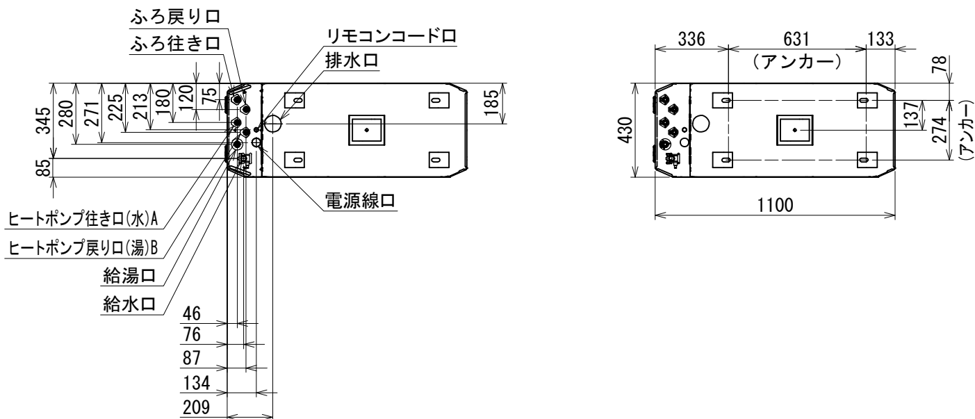
【配管位置上面透視図】
