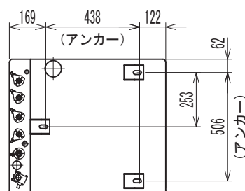
【アンカーボルト位置上面透視図】
