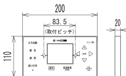
【ふろリモコン】 EBK-HFRG
