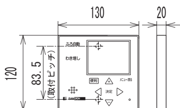
【増設リモコン】 EBK-ZRDG
