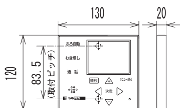
【台所リモコン】 EBK-HDRG
