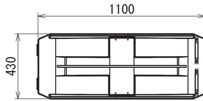
【機器側面図】
