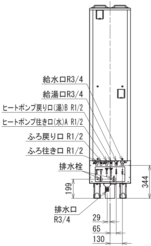
【機器正面図】
