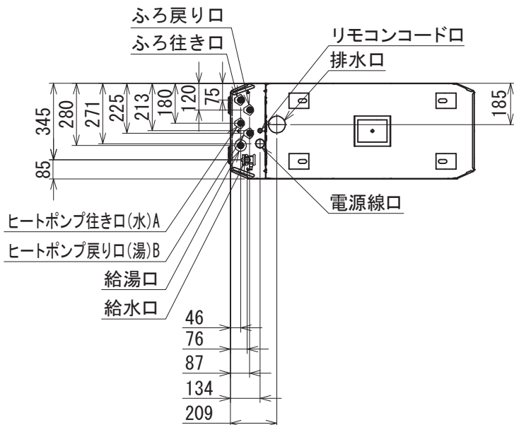
【配管位置上面透視図】
