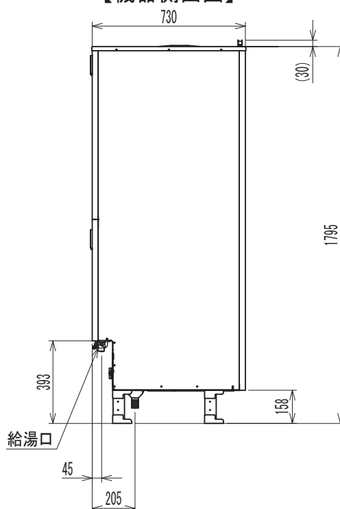
【機器側面図】
