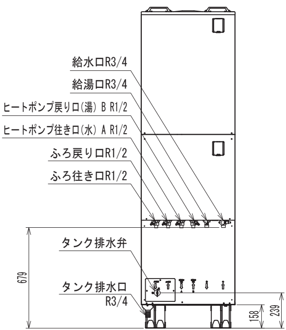
【機器正面図】
