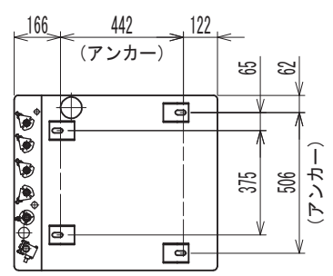
【アンカーボルト位置図(上面透視図)】
