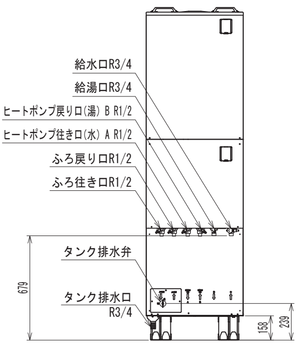
【機器正面図】
