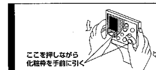
図10 化粧枠の取り外しかた
