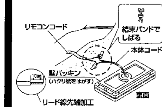
図2 閉端接続子によるコード圧着のしかた
