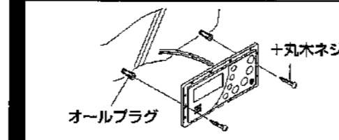
図3 リモコン本体の壁面への固定のしかた
