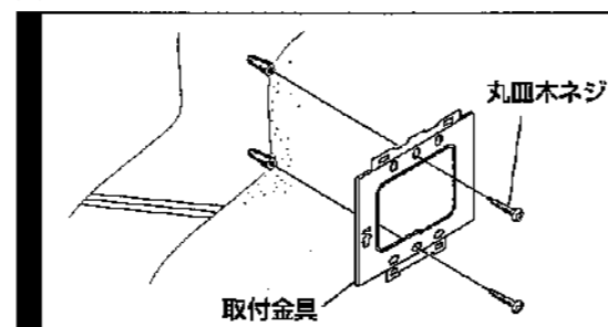
図3 コンクリート壁面への固定の場合
