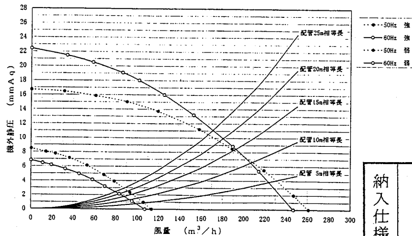
換気風量 - 静圧特性
