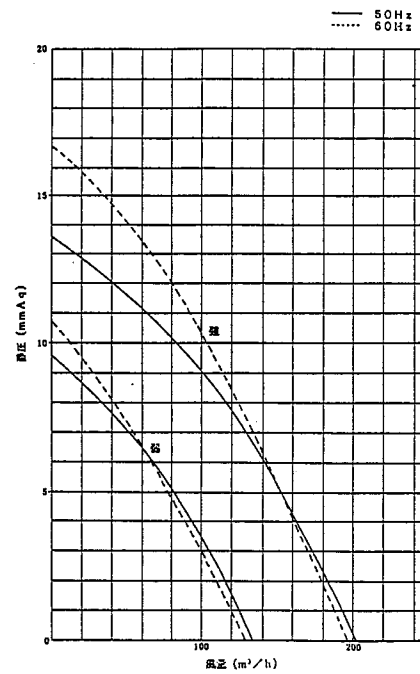
換気・静圧・風量特性曲線 (A 排気)
