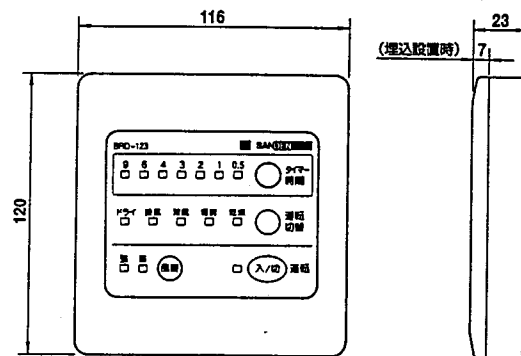
リモコン外形寸法図
