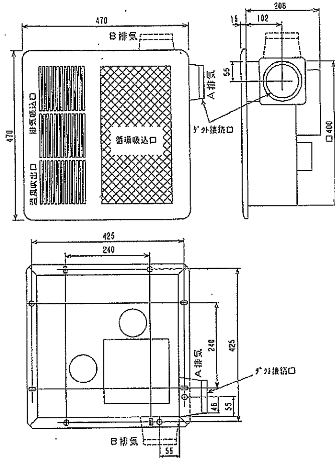
■ 本体寸法図
