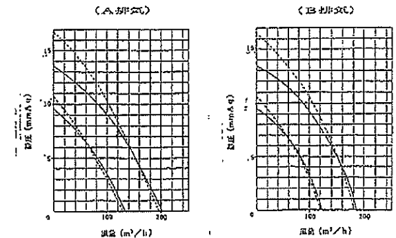
換気・暖房・乾燥性能曲線
