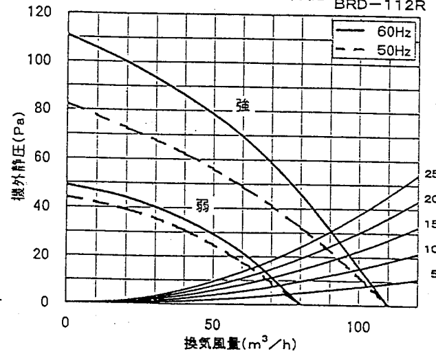
換気風量・静圧特性 BRD-112R
