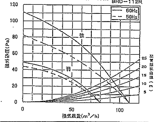
換気風量・静圧特性 BRD-112R
