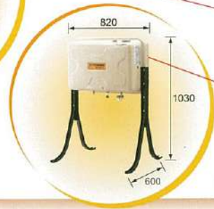
屋外油タンク FT-905 (90L) メーカー希望小売価格 ¥25,200 (税抜き価格 ¥24,000)
