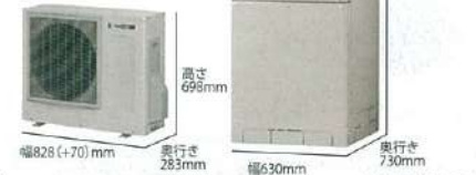
※写真はEBS-AHP46QTA ※写真は別売の配管カバー付き。
